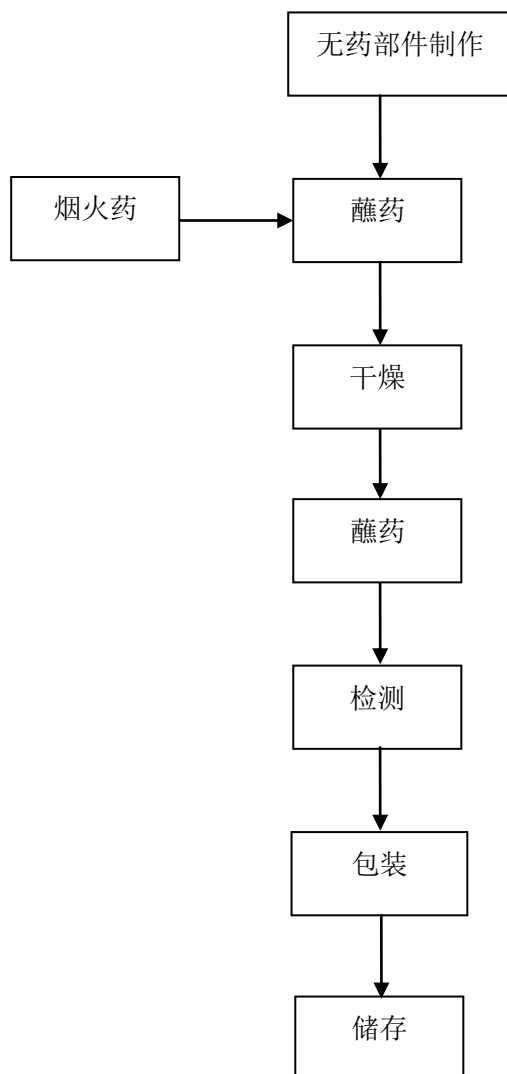
图A.22 电点火头生产流程图
