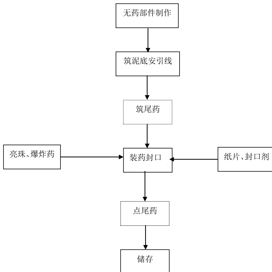
图A.5 效果内筒生产工艺流程
