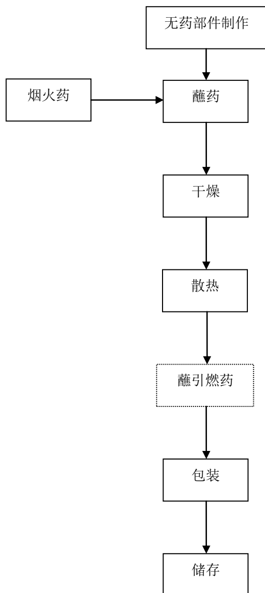
图A.14 线香类（涂敷型）生产流程图
