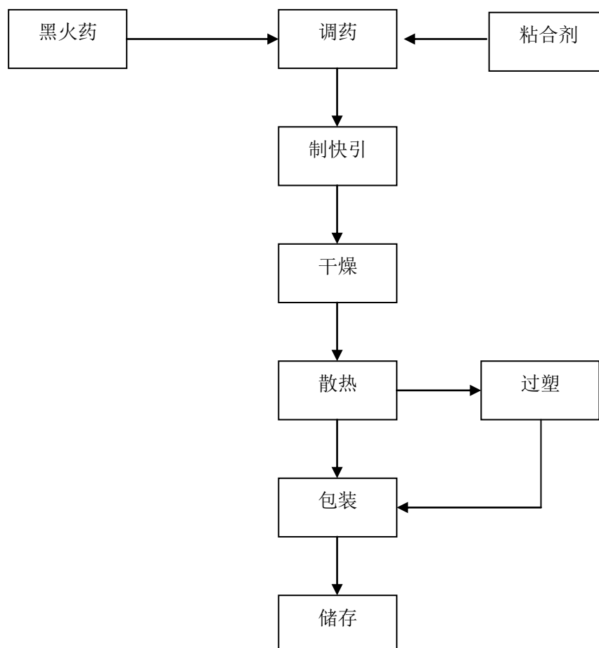
图A.4 皮纸快引生产工艺流程图
