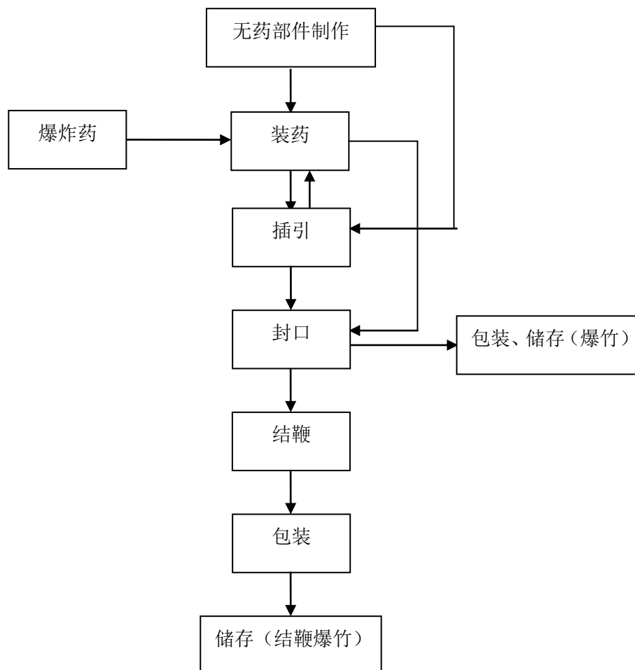
图A.12 结鞭类爆竹生产流程图
